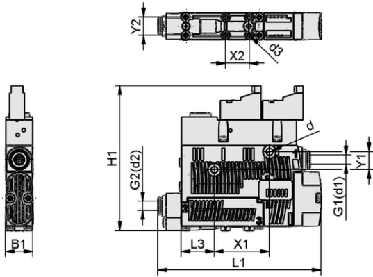
Tasarım verileri SCPSb 2-07 S04 NO
