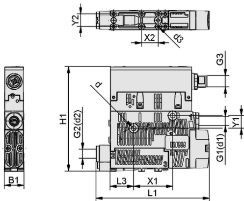
Données de construction SCPSi 2-14 G02 NO M12-5
