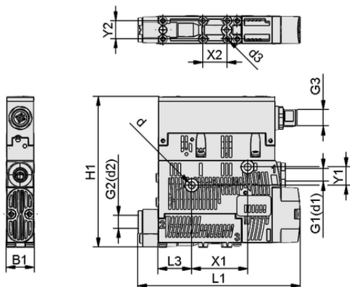
Dati di costruzione SCPS 2-07 G02 NC M12-5 PNP
