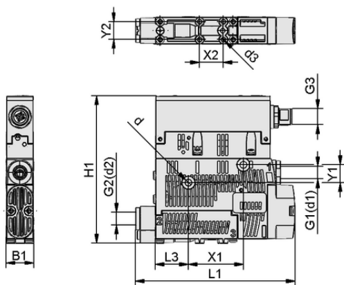
Données de construction SCPS 2-07 G02 NC M12-5 PNP
