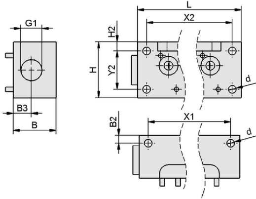
Tasarım verileri GP 4 SCPS 07..15 G2
