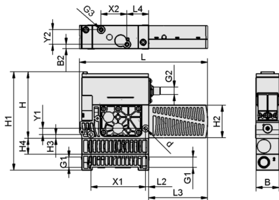
Dati di costruzione SXMPi 25 NC H PC M12-8
