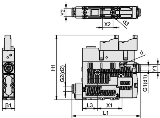
Données de construction SCPSb 15 S02 NC
