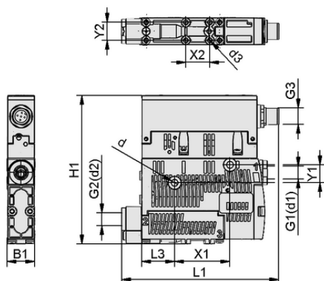
Dati di costruzione SCPSi 15 G02 NC M12-5
