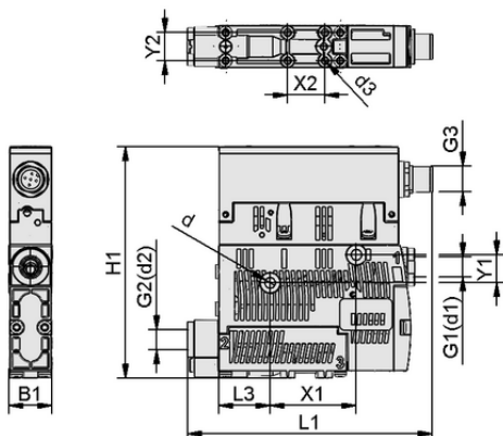
Dati di costruzione SCPSi 15 G02 NO M12-5
