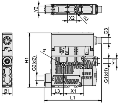
Tasarım verileri SCPSi 15 G02 NO M12-5
