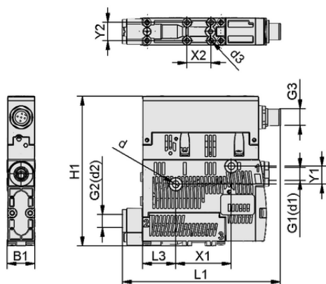
Données de construction SCPSi 15 G02 NO M12-5
