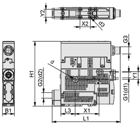
Dati di costruzione SCPS 07 G02 NC M12-5 PNP
