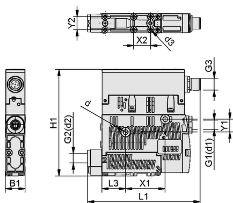
Données de construction SCPS 07 G02 NO M12-5 PNP
