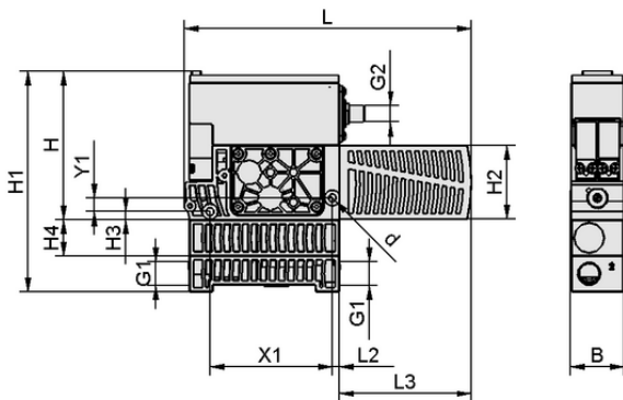
Données de construction SXMPi 30 IMP H PC 2xM12-5
