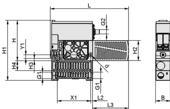
Dati di costruzione SXMPi 30 IMP H PC 2xM12-5
