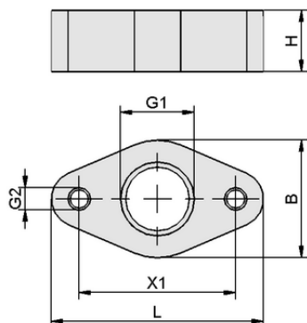
デザインデータ ADP-EJ 38x20x11-G1/8-IG SEAC
