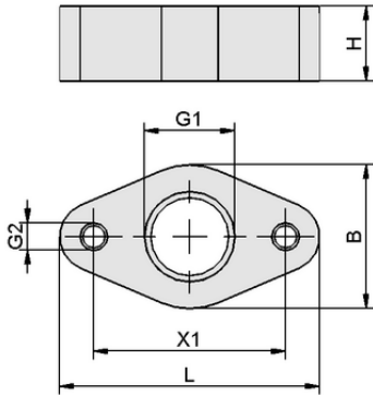
Tasarım verileri ADP-EJ 38x20x11-G1/4-IG SEAC
