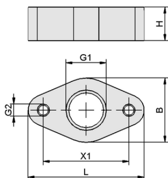
デザインデータ ADP-EJ 38x20x11-G1/4-IG SEAC
