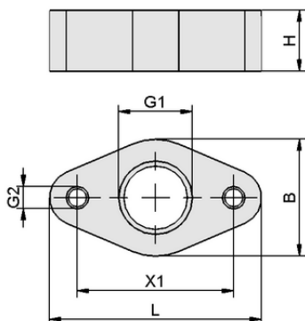
Dati di costruzione ADP-EJ 38x20x11-G1/4-IG SEAC
