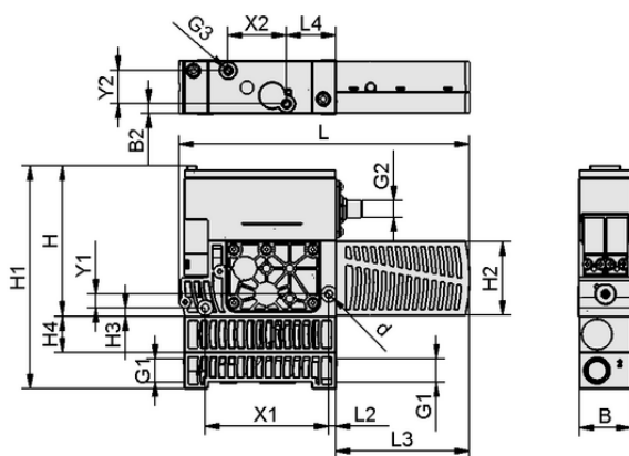
Dati di costruzione SXMPi 25 IMP H 2xM12-5
