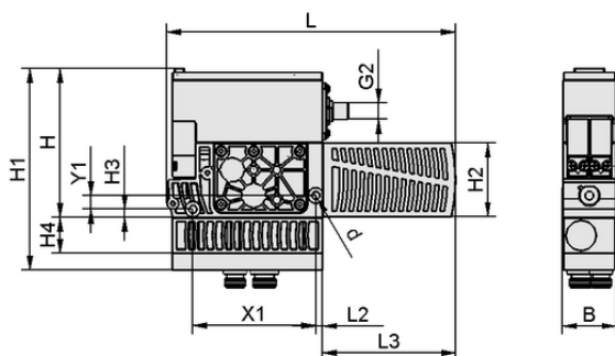
Dati di costruzione SXMPi 30 NO Q M12-8
