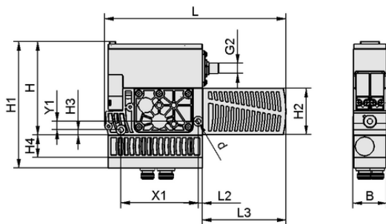
Dati di costruzione SXMPi 25 NO Q 2xM12-5
