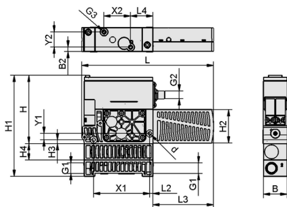
Dati di costruzione SXMPi 25 NO H M12-8
