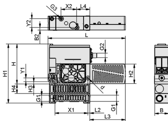
Dati di costruzione SXPi 25 IMP H 2xM12-5
