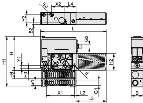
Données de construction SXPi 25 IMP H M12-8
