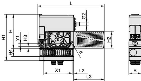
Données de construction SXPi 30 NC Q 2xM12-5
