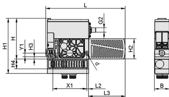
Dati di costruzione SXPi 30 NC Q 2xM12-5
