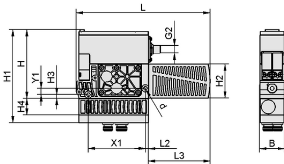
Données de construction SXPi 25 NC Q 2xM12-5
