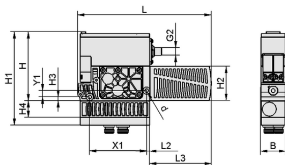
Données de construction SXPi 30 NO Q 2xM12-5
