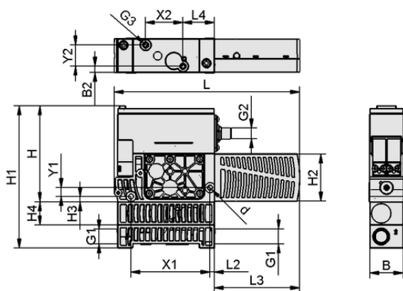
Dati di costruzione SXPi 30 NO H 2xM12-5
