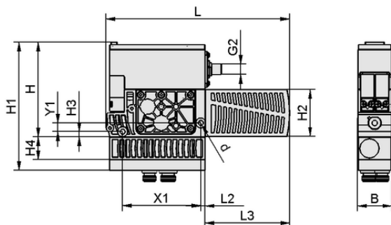
Dati di costruzione SXPi 25 NO Q 2xM12-5
