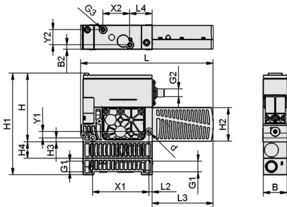
Données de construction SXPi 25 NO H M12-8
