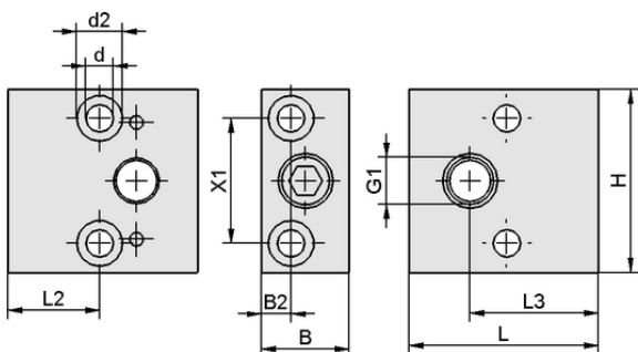
デザインデータ ADP-EJ 45.5x21x44-G1/4-IG SEAC VA-L
