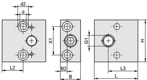
Dati di costruzione ADP-EJ 45.5x21x44-G1/4-IG SEAC VA-L
