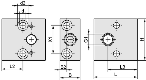
Tasarım verileri ADP-EJ 45.5x21x44-G1/4-IG SEAC VA-L
