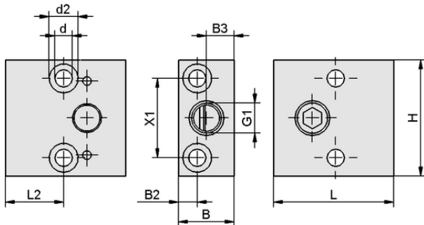
デザインデータ ADP-EJ 45.5x21x44-G1/4-IG SEAC VA-S
