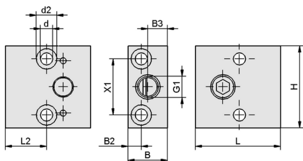
Dati di costruzione ADP-EJ 45.5x21x44-G1/4-IG SEAC VA-S
