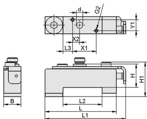
Données de construction ADP-Q 90.5x22x29.7 SMPi/SCPi
