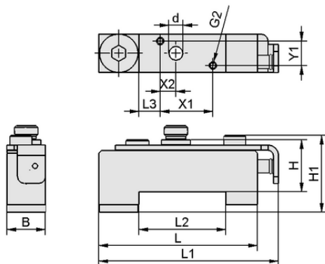
デザインデータ ADP-Q 90.5x22x29.7 SMPi/SCPi
