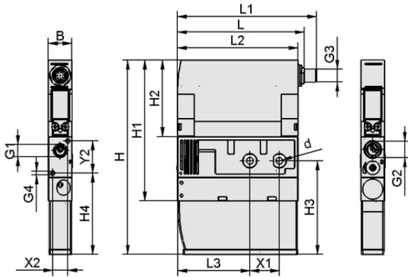
Tasarım verileri SCPi 20 NC VD M12-5
