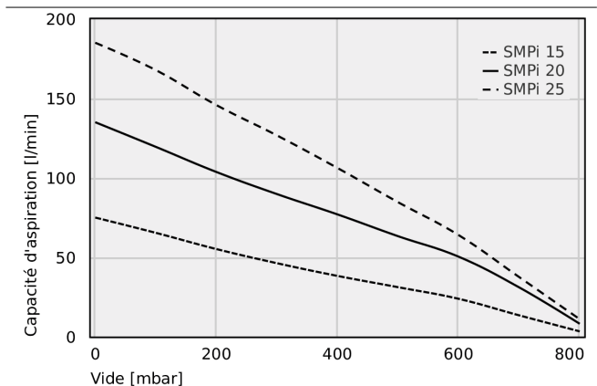
Capacité d'aspiration à différents degrés d'évacuation [l/min]
