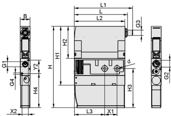
Données de construction SMPi 20 NC VD M12-5
