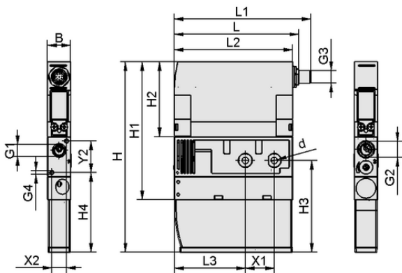
Données de construction SMPi 15 IMP RD M12-5
