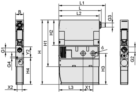
Tasarım verileri SMPi 15 NC RD M12-5
