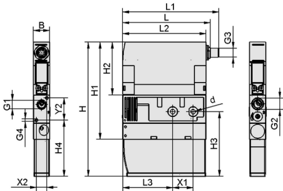
Données de construction SMPi 15 NC RD M12-5
