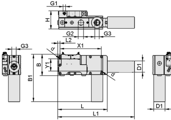
Tasarım verileri SEM-C 100 SDA NO AS
