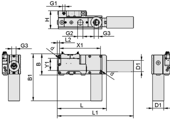
Tasarım verileri SEM-C 50 SDA NO AS
