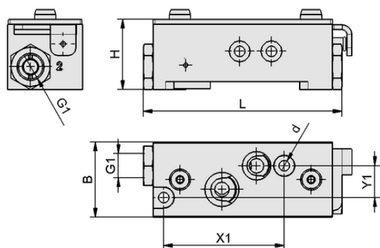
デザインデータ GPQ1 122x46x43 SXPi/SXMPi
