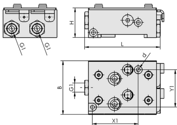
Données de construction GPQ2 122x87x48 SXPi/SXMPi
