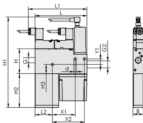
Dati di costruzione SCP 20 NO AS RP
